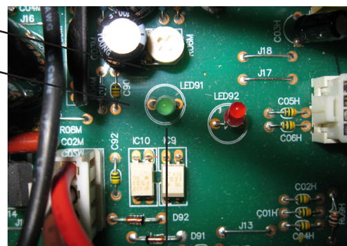
LED1 (Green)
